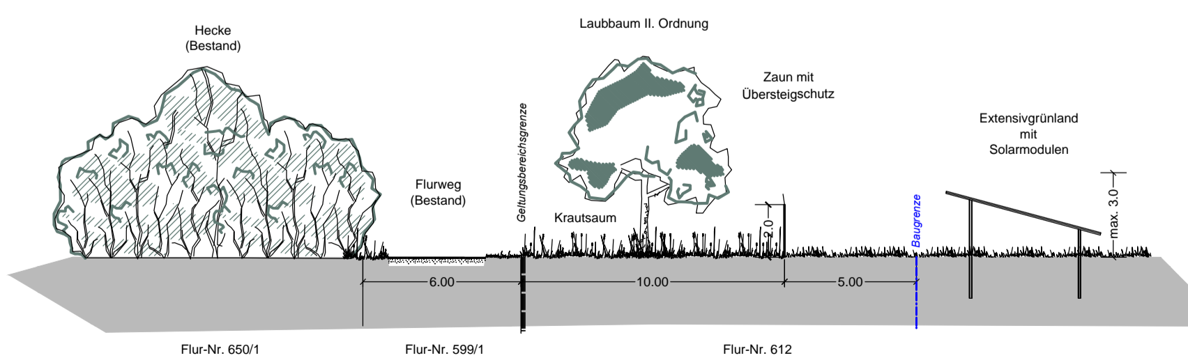
SCHNITT A - A' M 1:200
