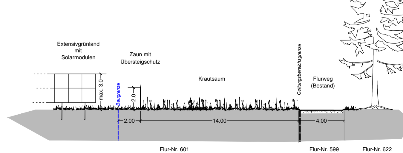
SCHNITT B - B' M 1:200
